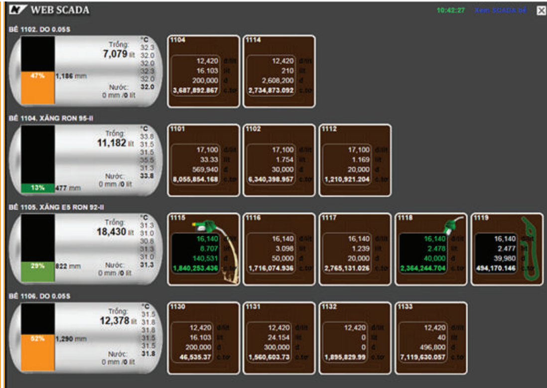
Màn hình SCADA theo dõi tình hình bán hàng qua cột bơm
